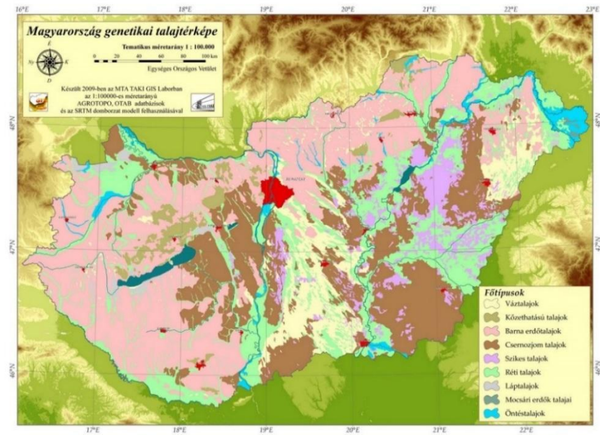
8. Ábra Talaj főtipusok
