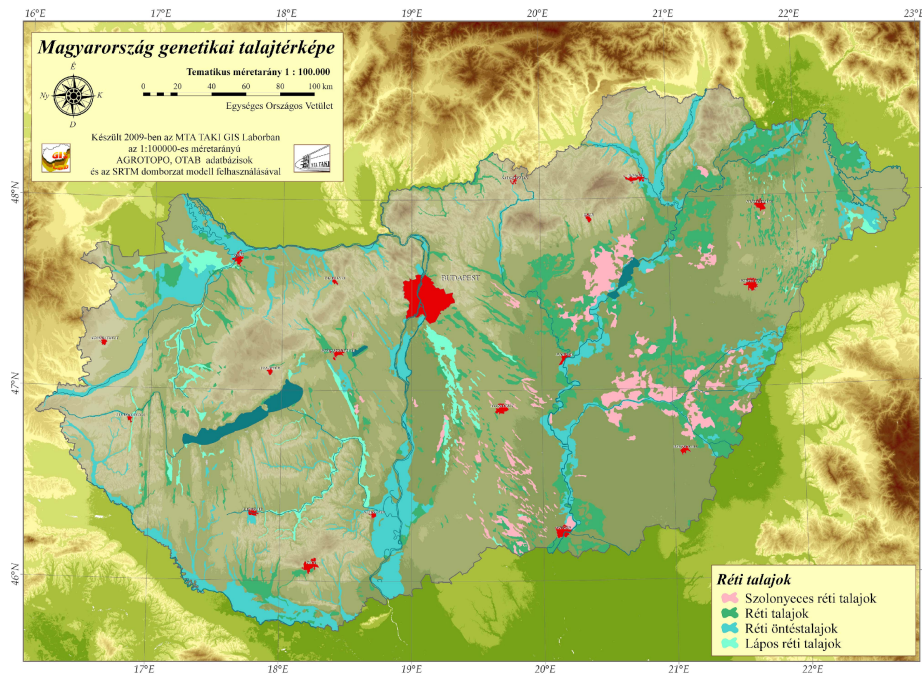
9. Ábra Réti talajok
