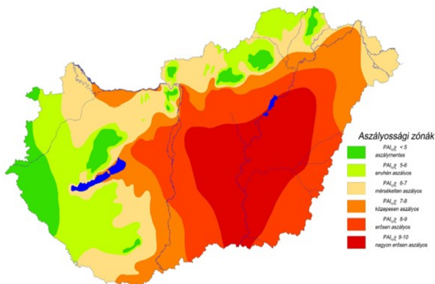
7. Ábra: PAI (Pálfai-féle aszályossági index)
